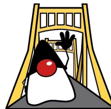
OrlandoJUG
