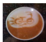
OrlandoJUG
